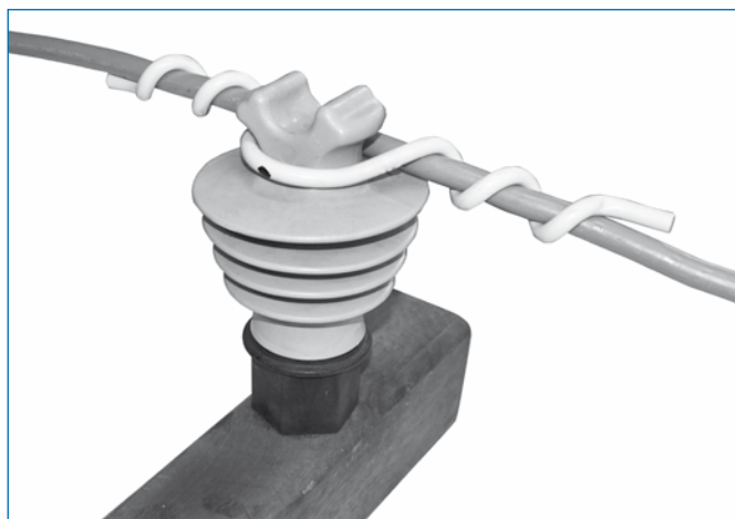
Isolador de Pino Ø pescoço = 57 mm
