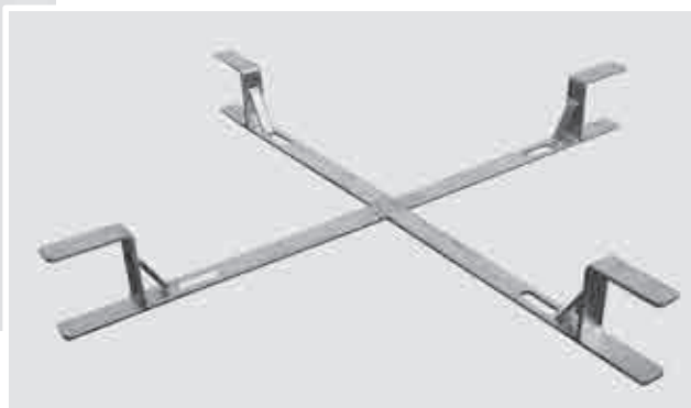
A fixação no montante da torre pode ser feita através de Suportes de Fixação à Compressão com Chapas em “L” ou com Garras.
