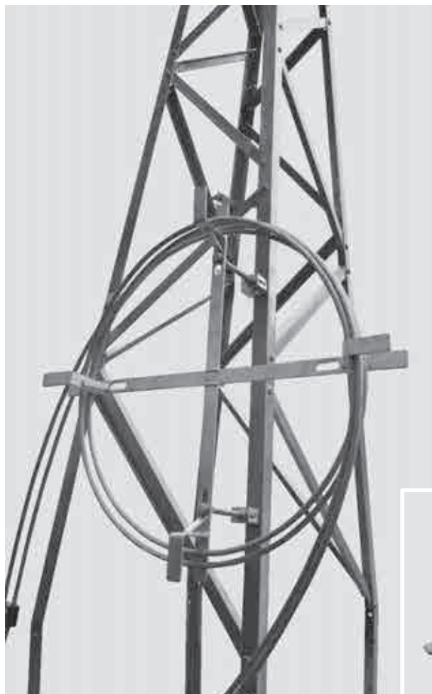
A fixação no montante da torre pode ser feita através de Suportes de Fixação à Compressão com Chapas em “L” ou com Garras.
