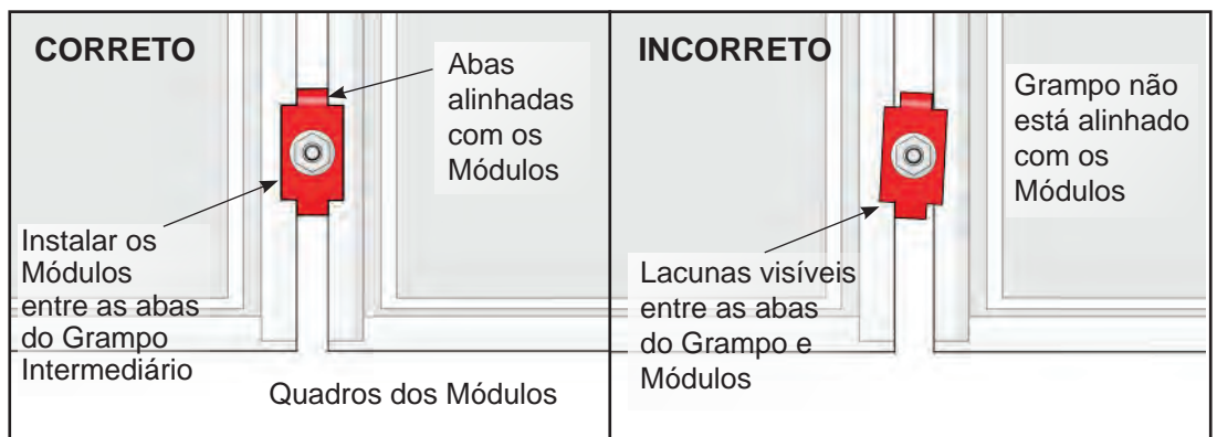
Figura 2: Métodos correto e incorreto de instalação padrão do Grampo Intermediário
