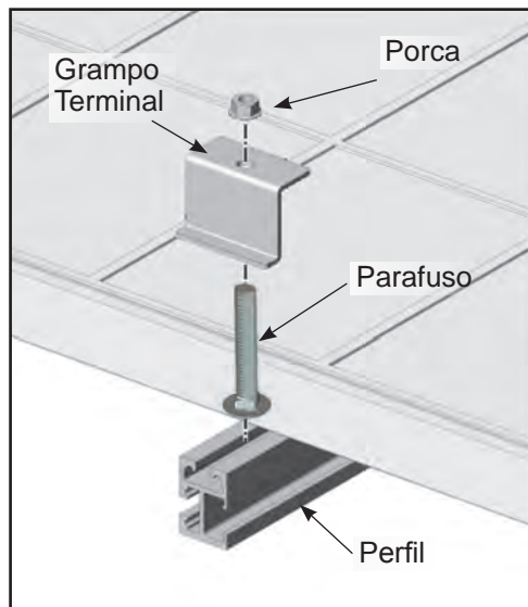
Figura 3: Instalando os Módulos utilizando Grampos Terminais
